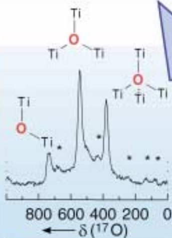
17 O-MAS-NMR Integrität des Ti-Oxo-Bausteins
