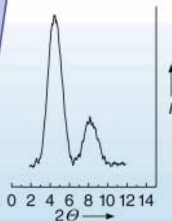
XRD Mesostruktur
