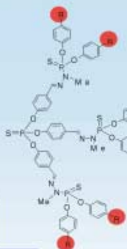
Dendrimer
